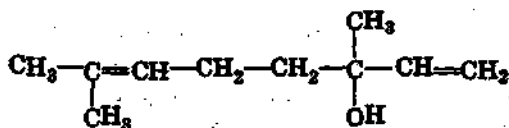
линалиол
