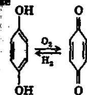
гидрохинон п-бензохинон
