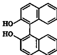
2,2'-дихокси-1,1'-бинафтали
