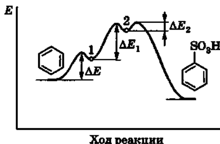
Рис. 60. Энергетические изменения при реакции электрофильного замещения в ароматическом ряду
