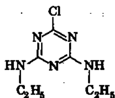
симазин
