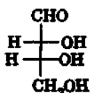
D (-) эритроза
