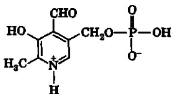
кодекарбоксилаза
