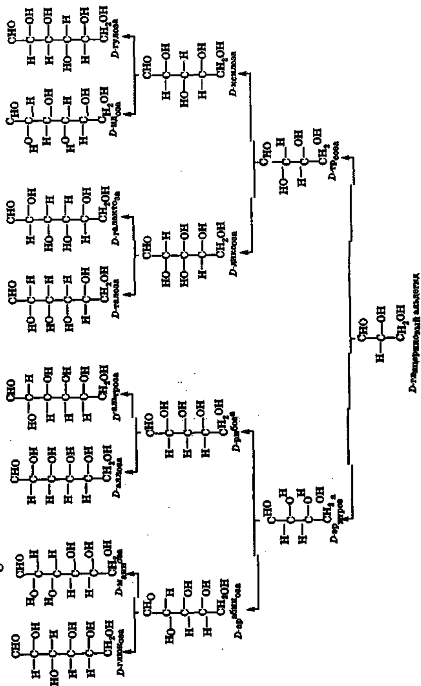
Схема 1. Генетический ряд D-глицеринового альдегида
