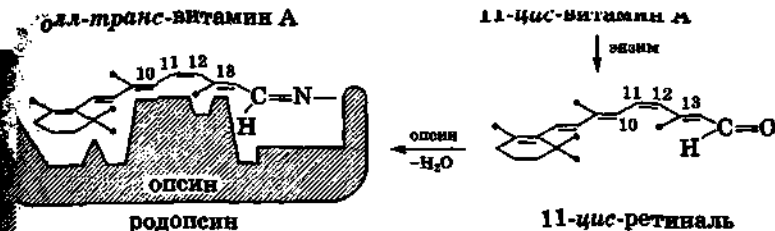
Рис. 65. Генетическая связь витамина А с родопсином
