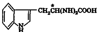
триптофан
