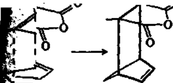
эндо-аддукт
