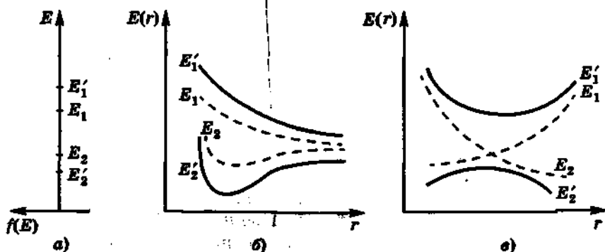
Рис. 16. Графическое изображение правила непересечения энергетических кривых одинаковых свойств симметрии
