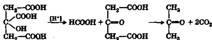
АЦЕТОНИКАРБОНОВАЯ КИСЛОТА
