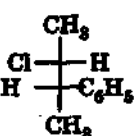
энантиомерные трео-2-хлор-3-фенилбутаны
