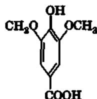
сиреневая кислота
