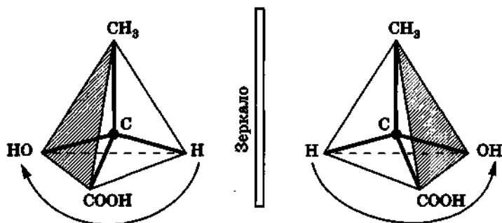
Рис. 75. Оптические изомеры
