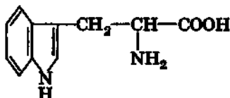
гетероциклическая аминокислота
