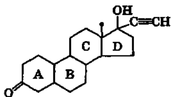
норэтидрон
