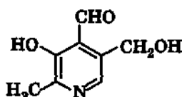
пиридоксаль
