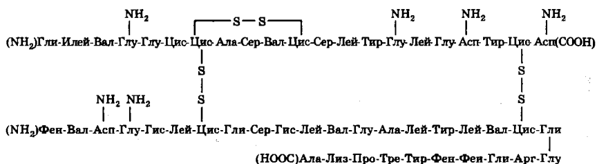
Рис. 86. Последовательность аминокислот в молекуле бычьего инсулина
