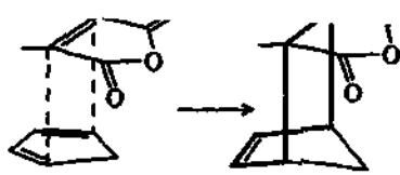
экзо-аддукт
