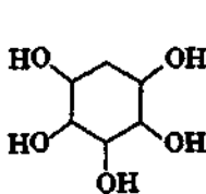
кверцит
