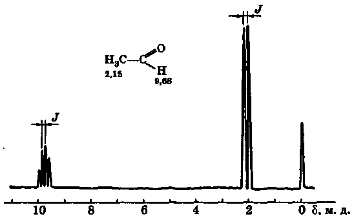
Рис. 70. ПМР-спектр ацетальдегида ( J = 2,8\text{ Гц} )
