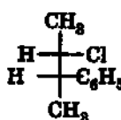
энантиомерные эритро-2-хлор-3-фенилбутаны
