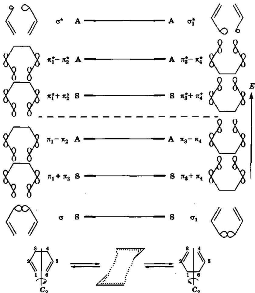
Рис. 54. Корреляционная диаграмма для сигматропной [3,3]-перегруппировки (перегруппировка Коупа)
