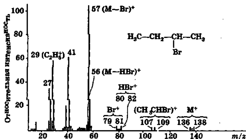
Рис. 51. Масс-спектр 2-бромбутана
