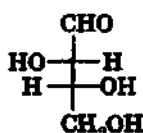
D (-) -треоза
