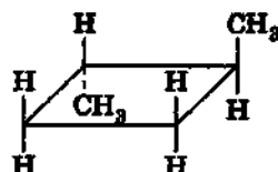
транс -1,2-диметилциклобутан
