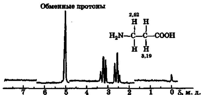
Рис. 83. ПМР-спектр \beta -аланина ( J = 9,0 \text{ Гц} )
