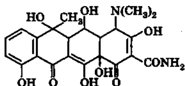
тетрациклин
