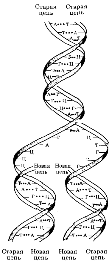
Рис. 93. Возможный механизм репликации ДНК
