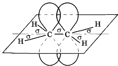
Рис. 19. Пространственное расположение орбиталей в молекуле этилена
