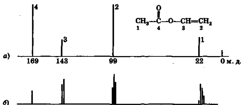
Рис. 46. Спектр ЯМР ^{13}\text{C} винилацетата:
