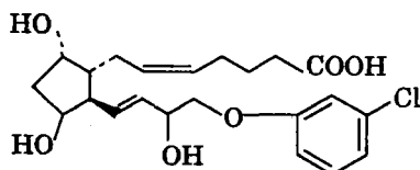
глопростенол
