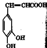
кофейная кислота
