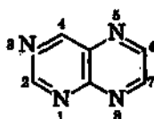
птеридин
