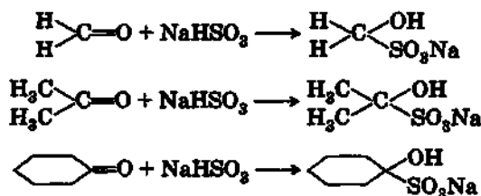
циклогексанон
