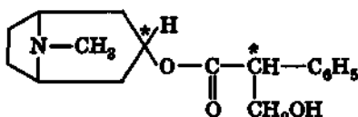
атропин
