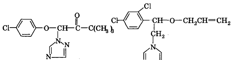
байлетон
