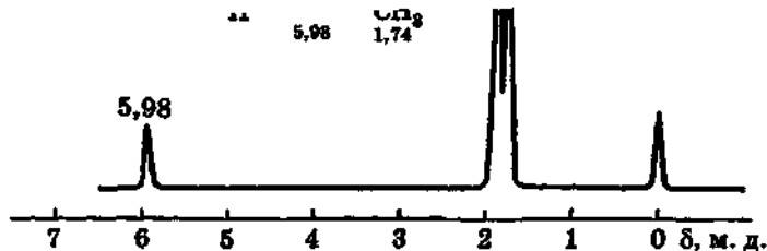
Рис. 57. ПМР-спектр сим-тетраметилбутадиена
