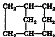
бицикло[3,2,1]октан
