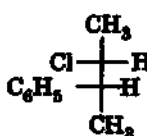
энантиомерные эритро-2-хлор-3-фенилбутаны
