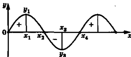
Рис. 1. Графическое изображение стоячей волны
