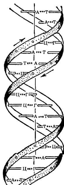
Рис. 92. Схематическое изображение двойной спирали ДНК
