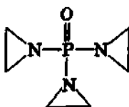
ТЭФА
