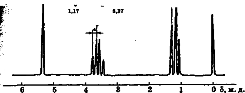
Рис. 67. ПМР-спектр этанола
