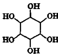
инозит
