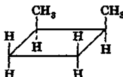
цис -1,2-диметилциклобутан
