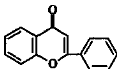
флавоны
