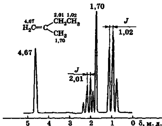
Рис. 55. ПМР-спектр 2-метилбутена-1 ( J = 7,2\text{ Гц} )
