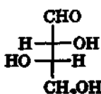
L (+) -треоза
