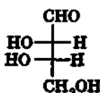
L (+) эритроза
