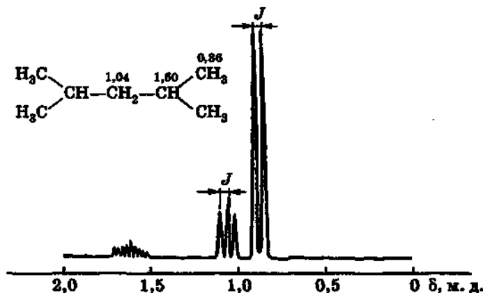
Рис. 53. ПМР-спектр 2,4-диметилпентана ( J = 7,6 \text{ Гц} )
