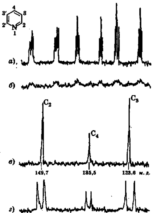
Рис. 45. Спектр ЯМР ^{13}\text{C} пиридина без двойного резонанса:
