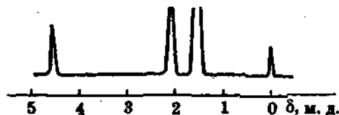
Рис. 64. ПМР-спектр метиленициклогексана
