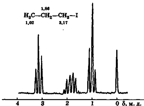
Рис. 66. ПМР-спектр 1-иодпропана
