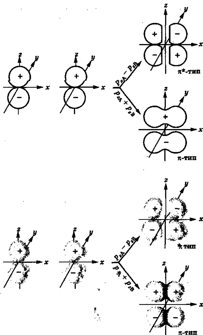
Рис. 12. Графическое изображение образования \pi - и \pi^* -орбиталей
